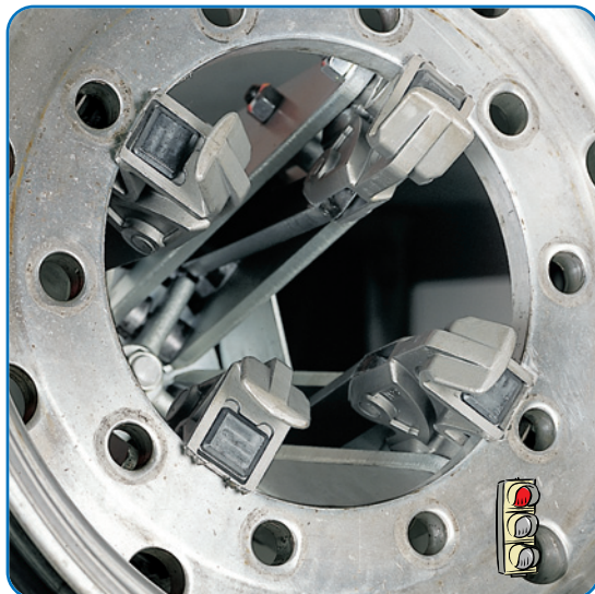
➤ Falsche Aufspannung. Direkter Kontakt mit der Spannklaue. Die Felge wird in jedem Fall beschädigt
