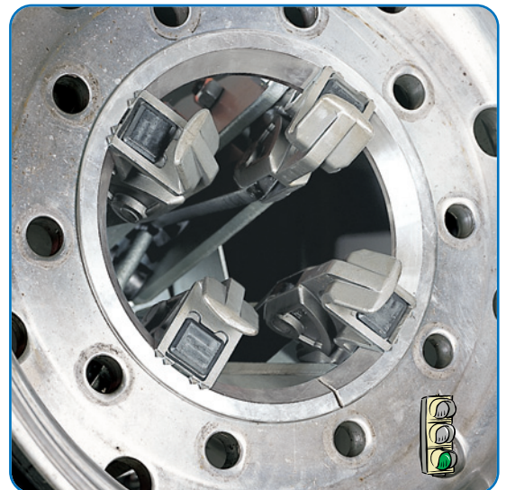
➤ Richtige Aufspannung mit Spannring. Kein direkter Kontakt zwischen Felge und Spannklaue. Maximale Schonung der Felge
